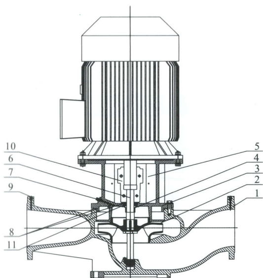
截面图TD200~TD250
