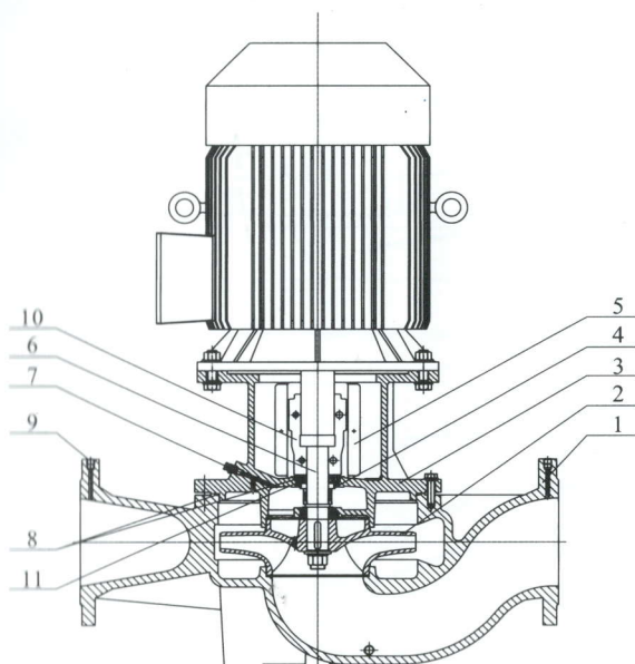
截面图TD125-18/4~TD150-50/4
