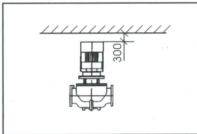
电机功率 < 5.5 kW泵的安装
